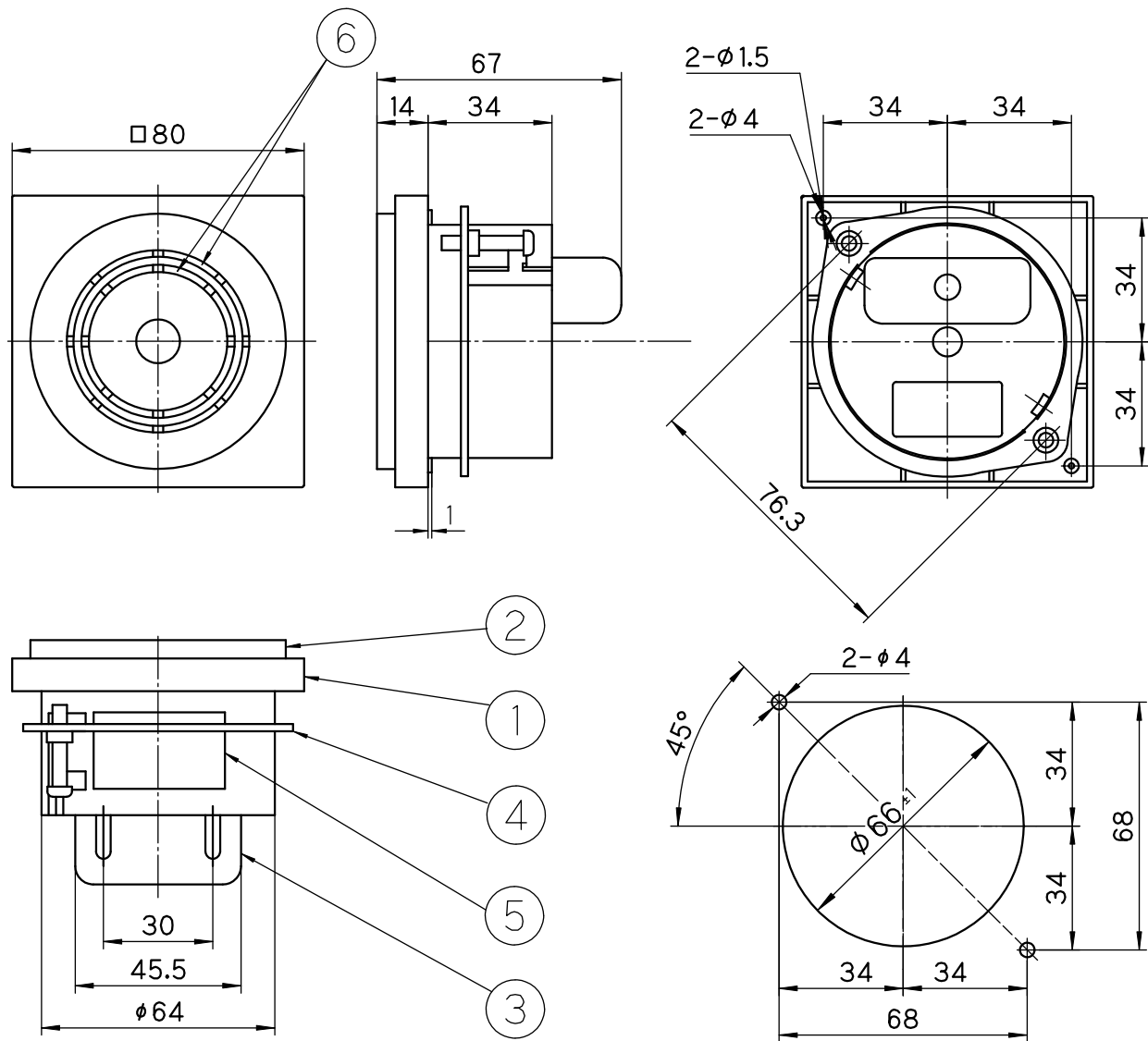
BZ-30板金加工寸法
