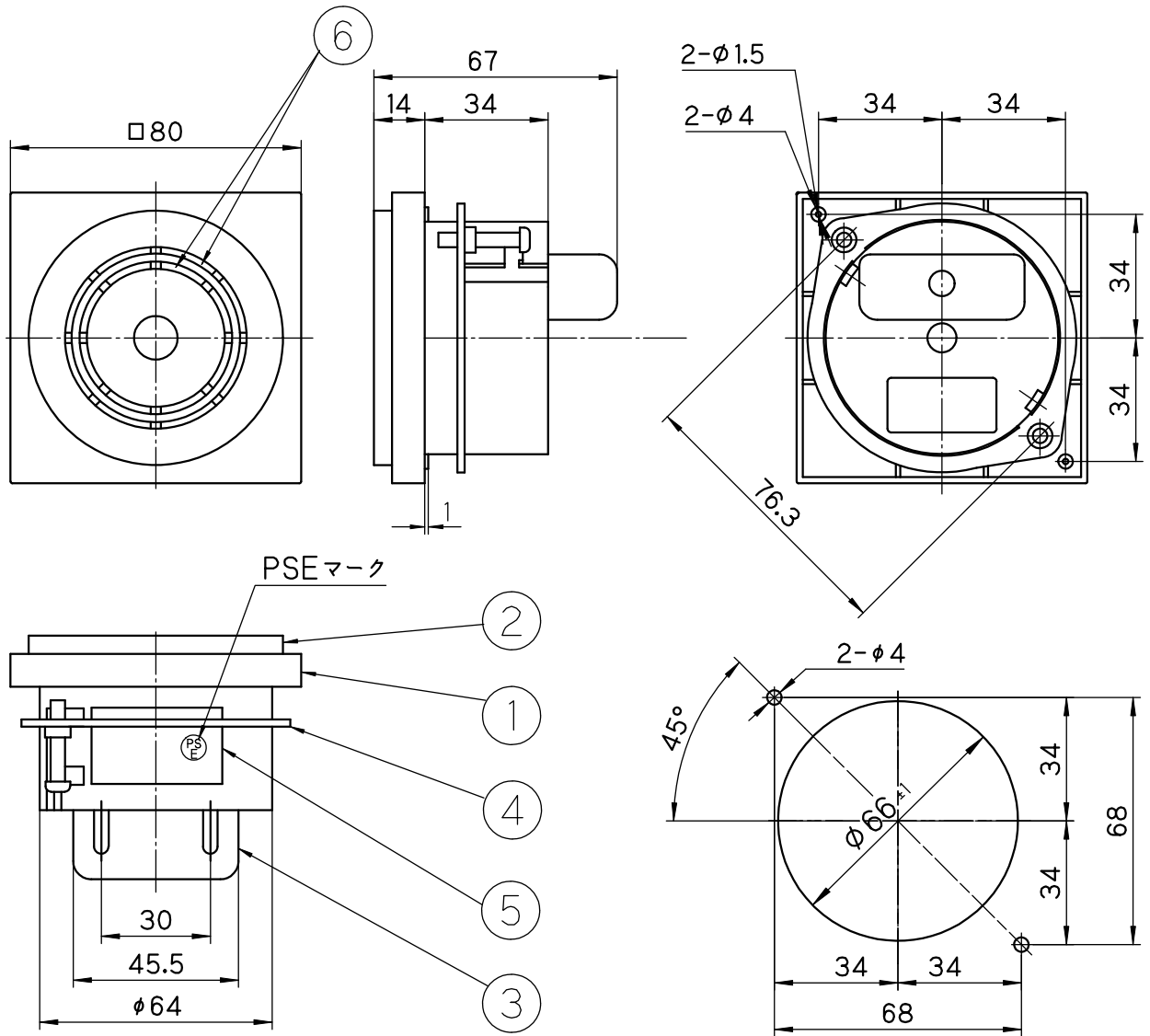
BZ-30板金加工寸法
